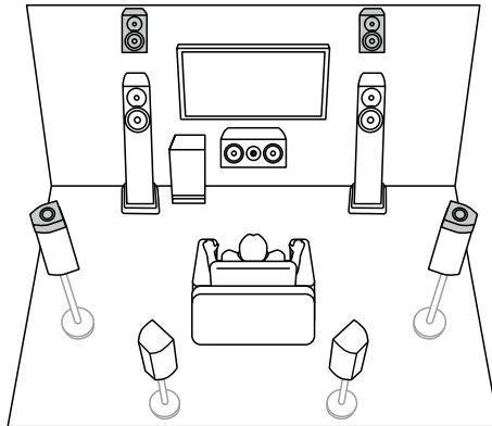
7.1.4チャンネル (フロントハイと Dolby Enabled スピーカー (サラウンド)) (→p33)
