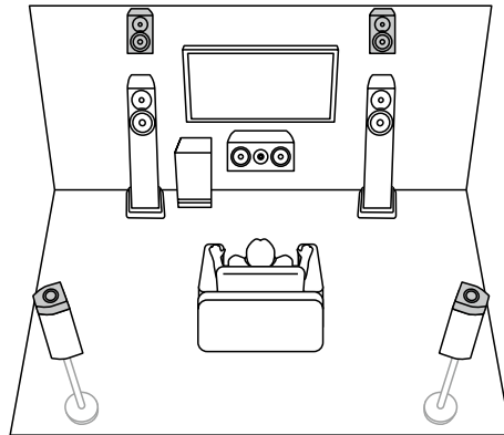
5.1.4チャンネル (フロントハイ と Dolby Enabled スピーカー (サラウンド)) (→p32)
