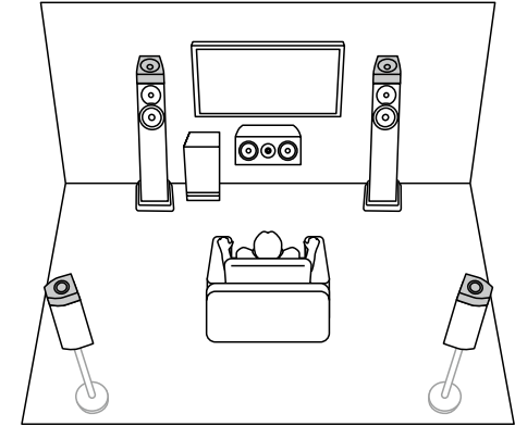
5.1.4チャンネル (Dolby Enabled スピーカー (フロント と サラウンド)) (→p32)
