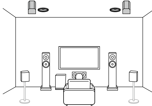
5.1.4チャンネル (トップミドル と リアハイ) (→p32)
