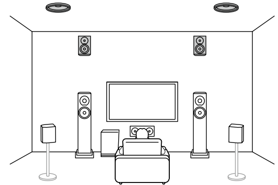
5.1.4チャンネル (フロントハイ と トップリア) (→p32)
